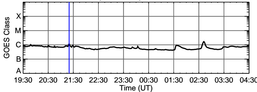
13-Feb-2011 (DOY 044) C1.1 @ 21:20:00 UT
