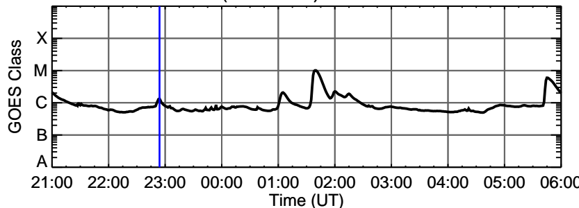
ESP 0-7 nm
