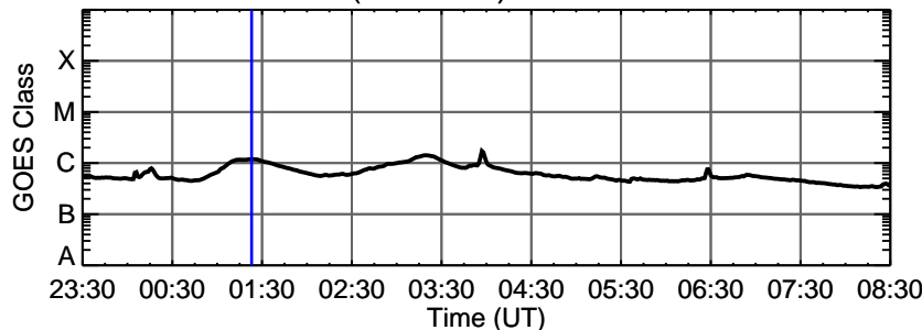
20-Feb-2011 (DOY 051) C1.2 @ 01:23:00 UT
