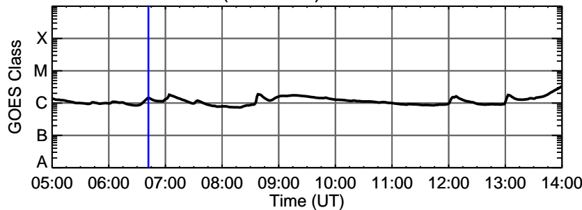
18-Nov-2013 (DOY 322) C1.4 @ 06:42:00 UT
