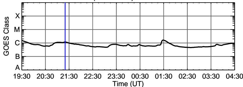
25-Nov-2013 (DOY 329) C1.1 @ 21:20:00 UT
