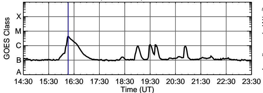
11-Nov-2010 (DOY 315) C4.3 @ 16:16:00 UT
