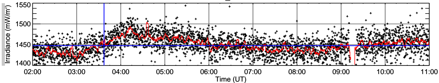
GOES-14 EUV-A
