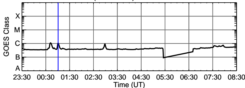
25-Mar-2011 (DOY 084) C1.0 @ 01:01:00 UT
