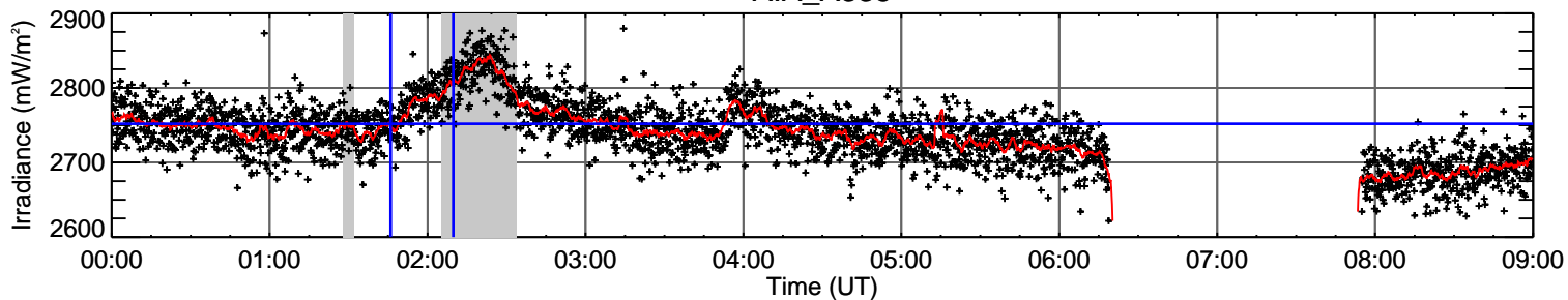
GOES-14 EUV-A
