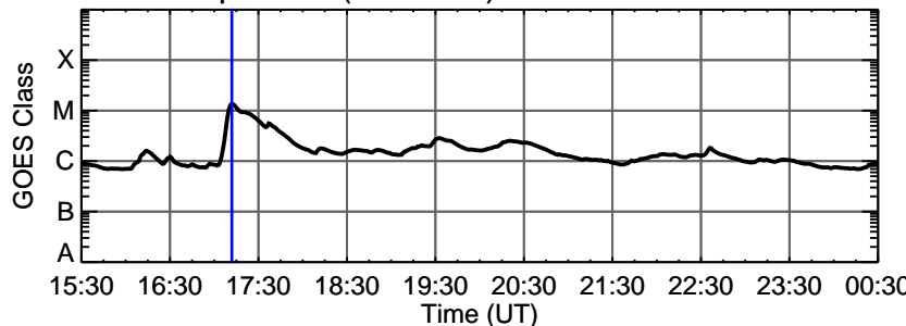
15-Apr-2011 (DOY 105) M1.3 @ 17:12:00 UT
