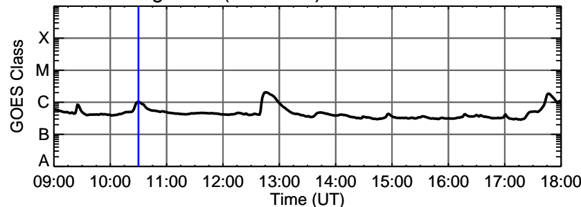
ESP 0-7 nm
