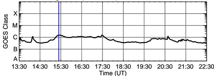
10-Aug-2011 (DOY 222) C1.5 @ 15:24:00 UT
