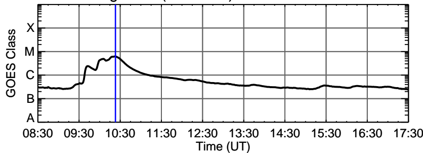
11-Aug-2011 (DOY 223) C6.2 @ 10:23:00 UT
