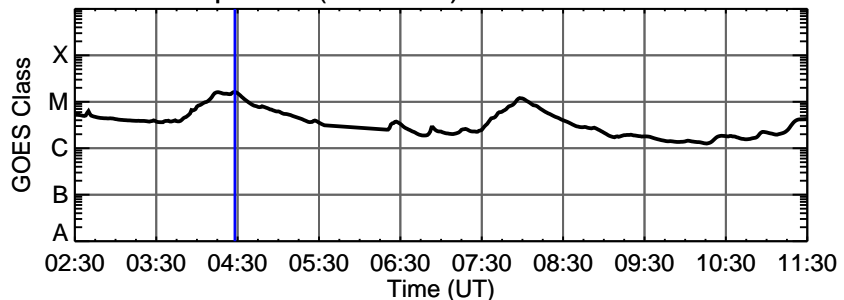
05-Sep-2011 (DOY 248) M1.6 @ 04:28:00 UT
