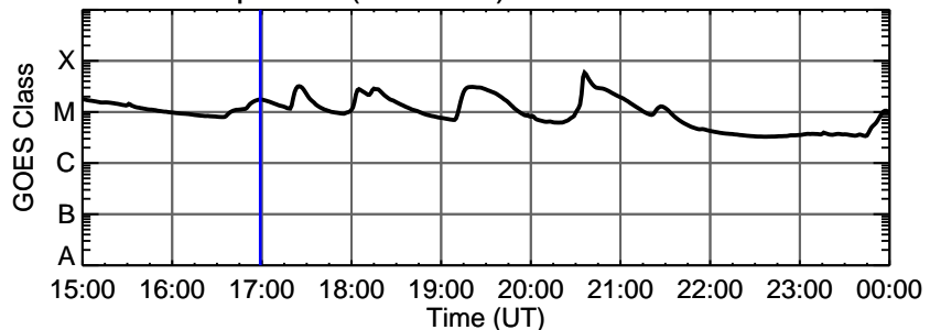
24-Sep-2011 (DOY 267) M1.7 @ 16:59:00 UT
