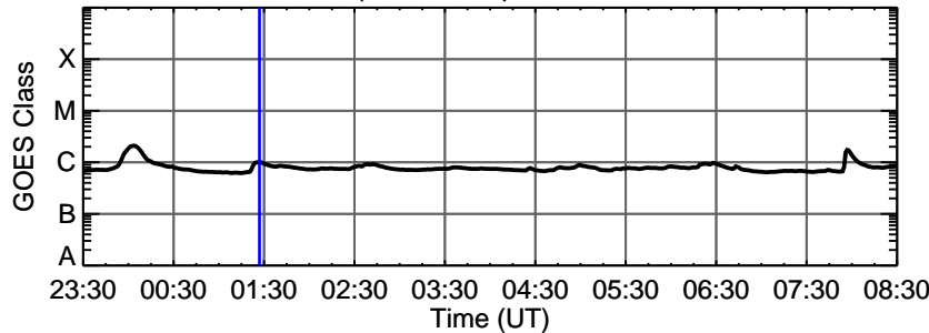
19-Nov-2011 (DOY 323) C1.0 @ 01:27:00 UT
