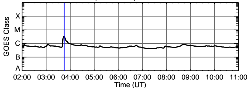
25-Nov-2011 (DOY 329) C3.3 @ 03:45:00 UT
