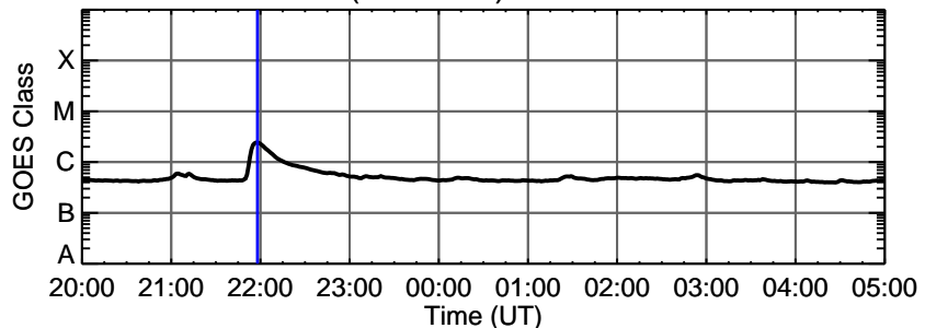
25-Nov-2011 (DOY 329) C2.4 @ 21:58:00 UT
