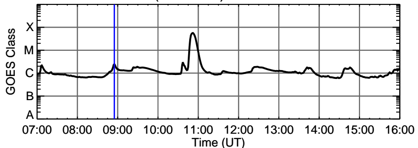
02-Jul-2012 (DOY 184) C2.4 @ 08:55:00 UT
