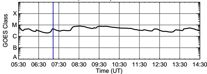
09-Jul-2012 (DOY 191) C4.5 @ 07:13:00 UT
