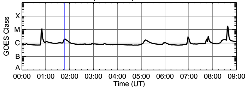
13-Jan-2013 (DOY 013) C1.9 @ 01:48:00 UT
