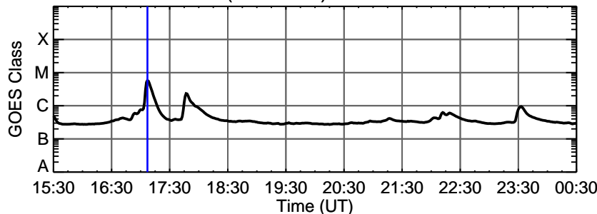
18-Jan-2013 (DOY 018) C5.8 @ 17:07:00 UT
