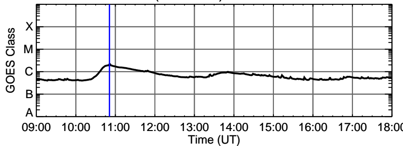
19-Feb-2013 (DOY 050) C2.1 @ 10:51:00 UT
