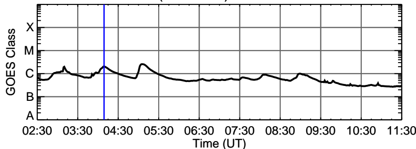
21-Feb-2013 (DOY 052) C2.0 @ 04:09:00 UT
