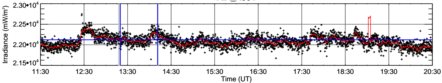
AIA_A335
