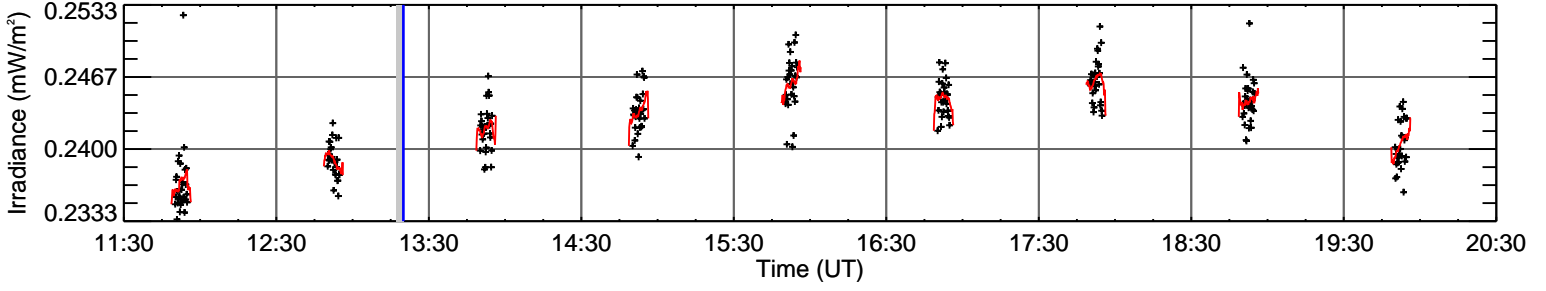
MEGS-B long
