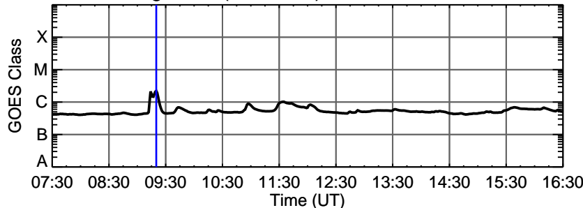
19-Aug-2013 (DOY 231) C2.2 @ 09:20:00 UT
