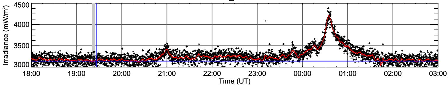
GOES-14 EUV-A
