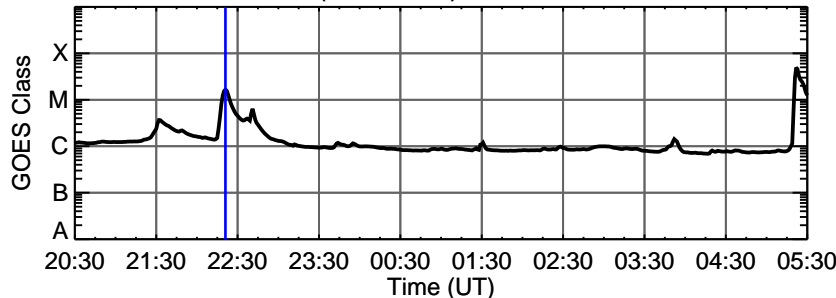
02-Nov-2013 (DOY 306) M1.6 @ 22:21:00 UT
