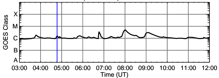
14-Nov-2013 (DOY 318) C1.5 @ 04:47:00 UT
