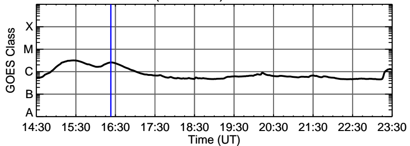
24-Nov-2013 (DOY 328) C2.5 @ 16:23:00 UT
