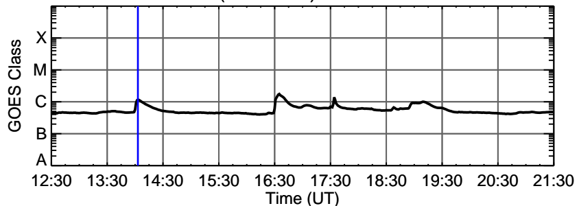
25-Dec-2013 (DOY 359) C1.1 @ 14:03:00 UT
