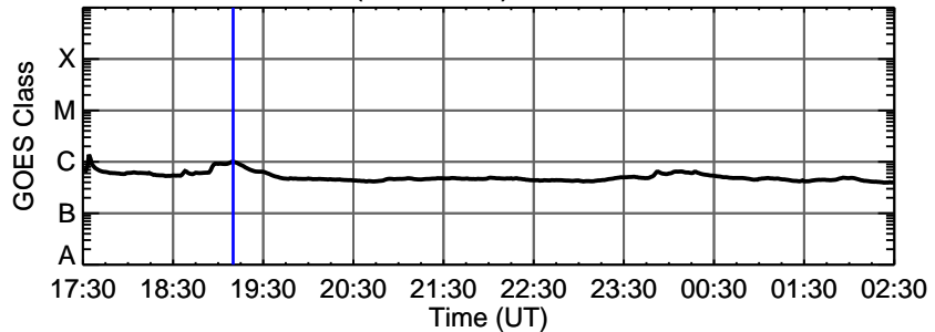
25-Dec-2013 (DOY 359) C1.0 @ 19:10:00 UT
