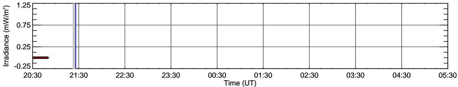
MEGS-B short
