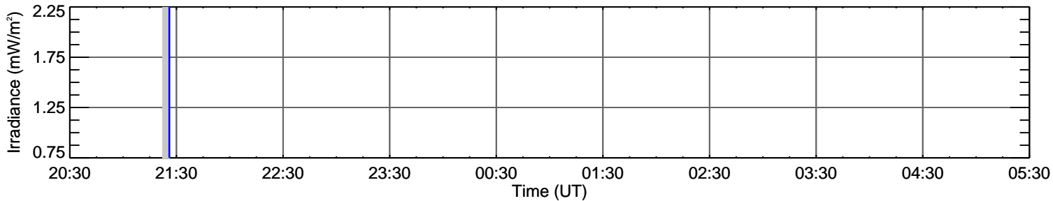
GOES-14 EUV-A
