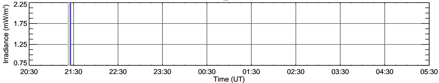
AIA_A211
