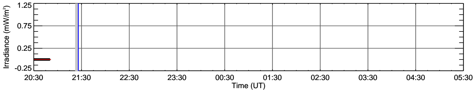
MEGS-A1
