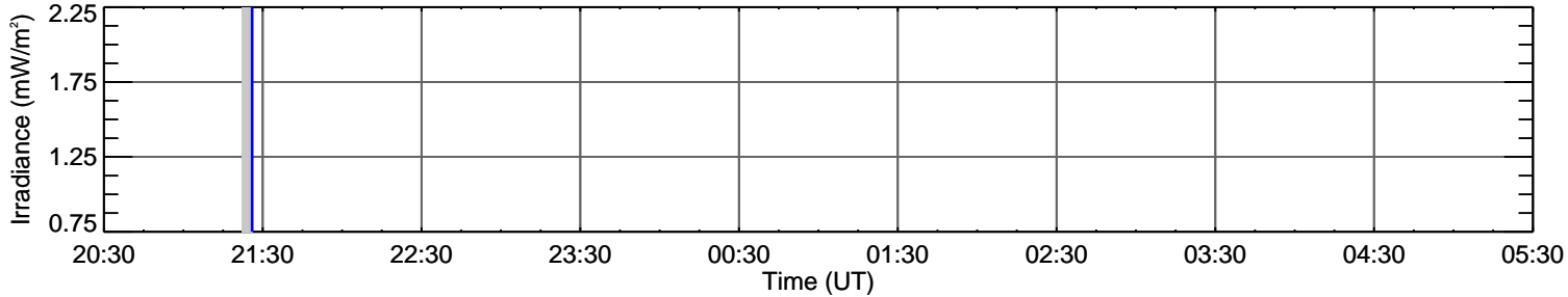
AIA_A335
