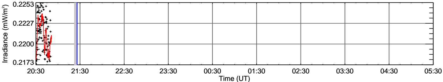
MEGS-B long
