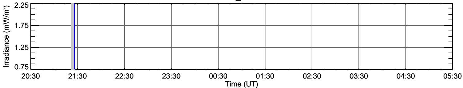
AIA_A304
