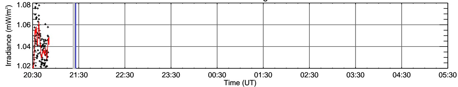
MEGS-B long
