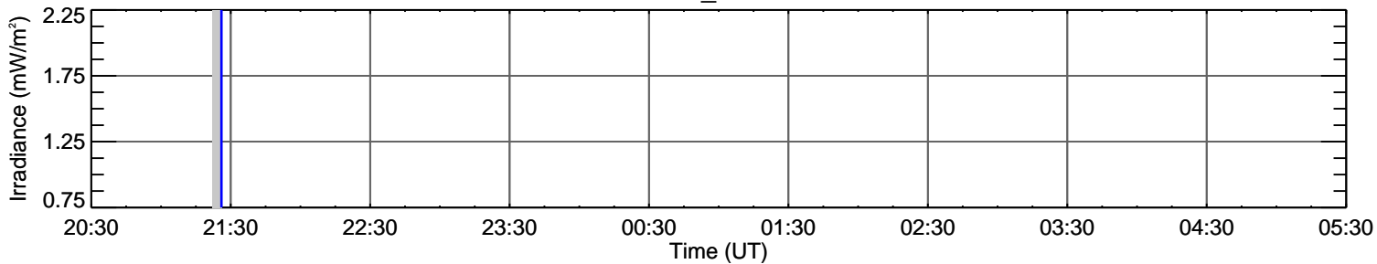
AIA_A193
