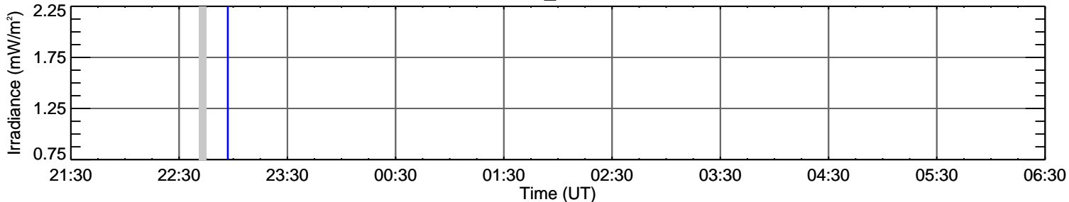
GOES-14 EUV-A
