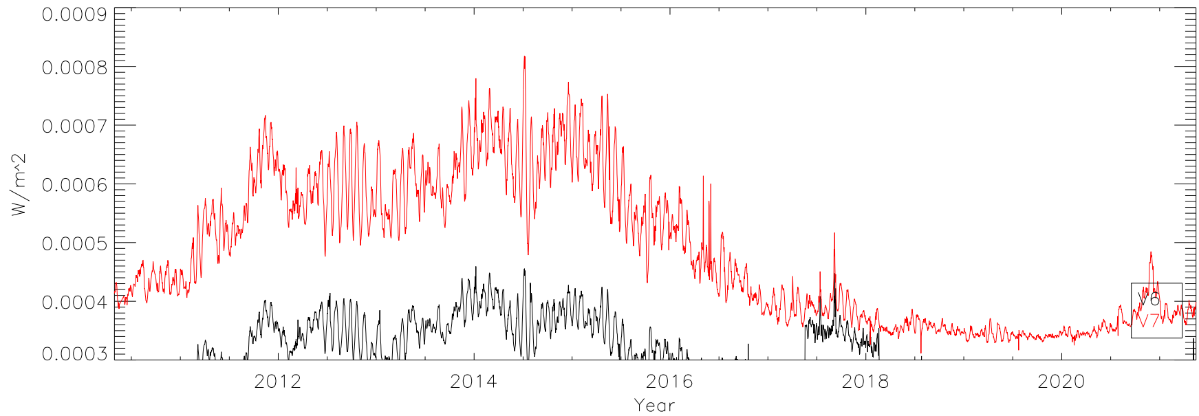
MEGS-B short
