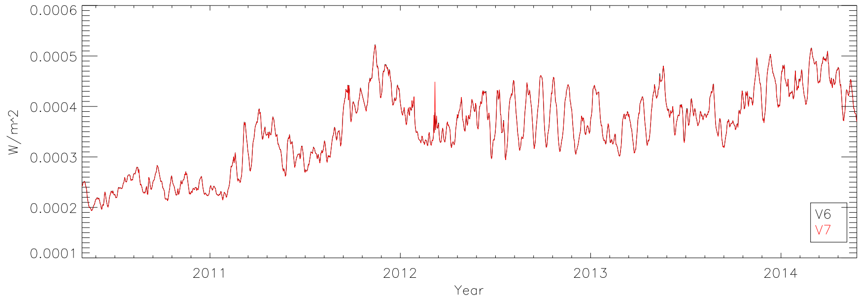
GOES-14 EUV-A
