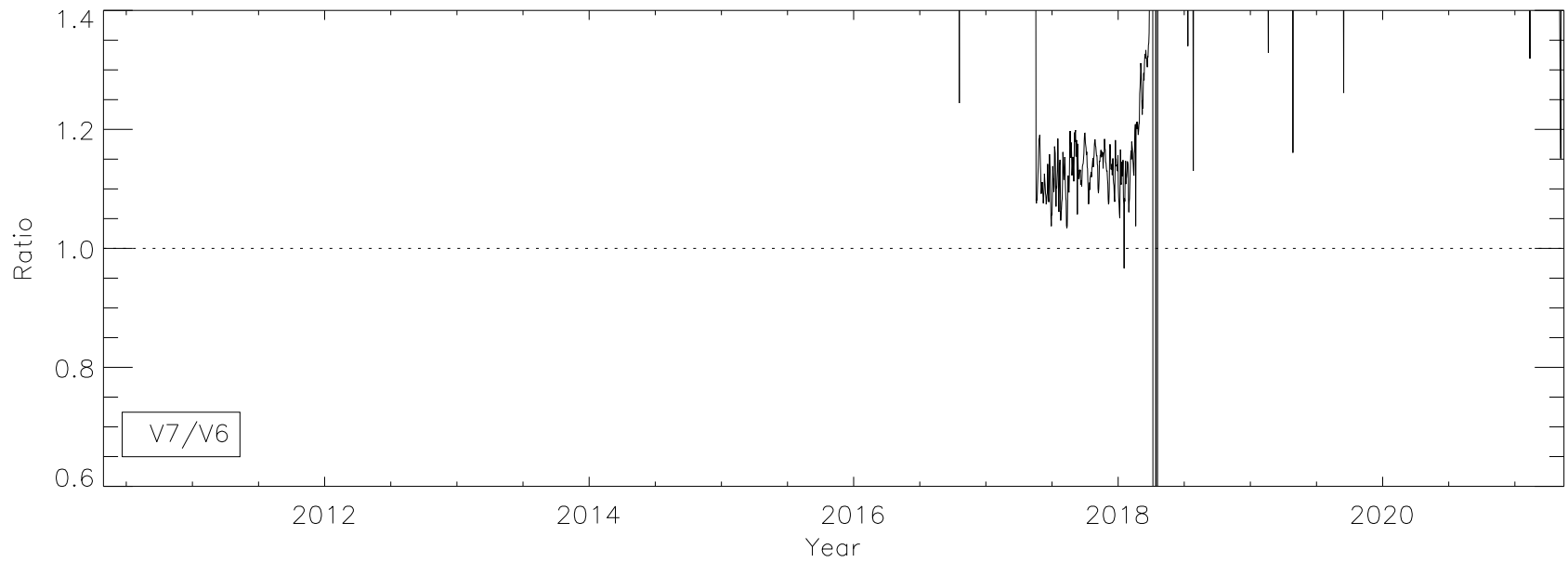
MEGS-B short
