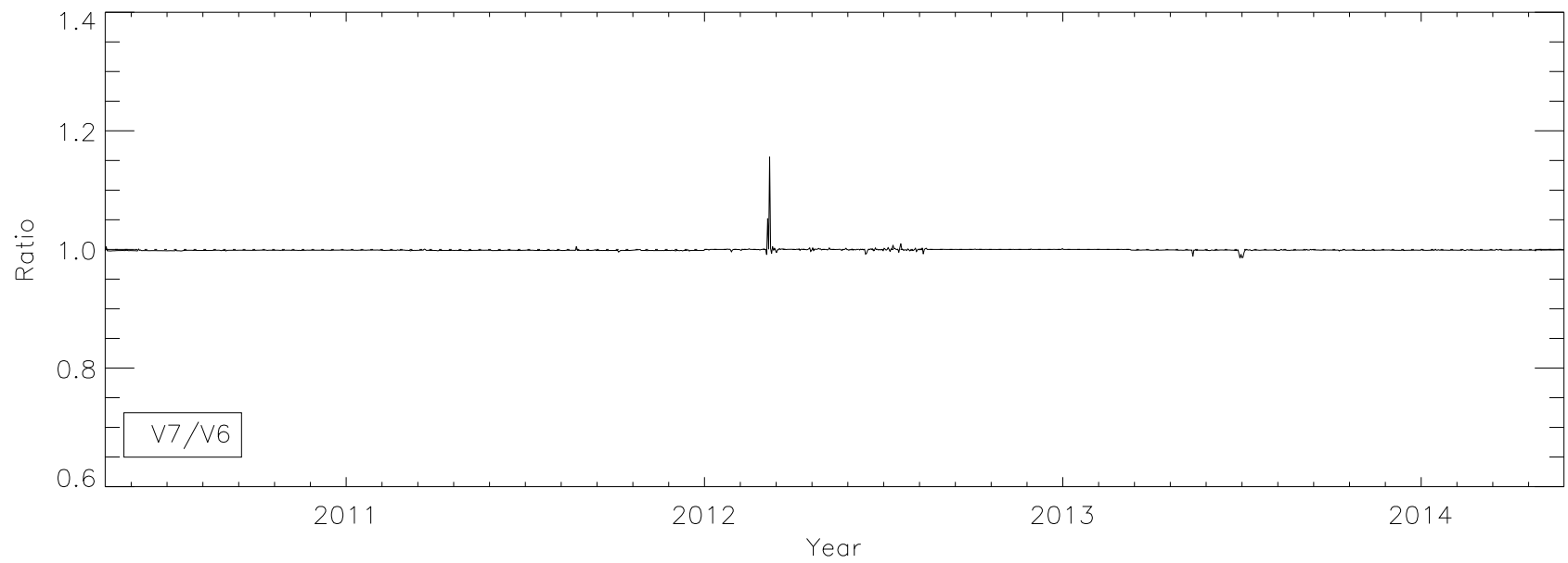
GOES-14 EUV-A
