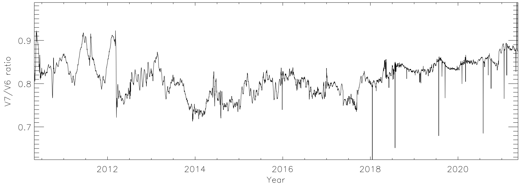
Ne VII 46.522
