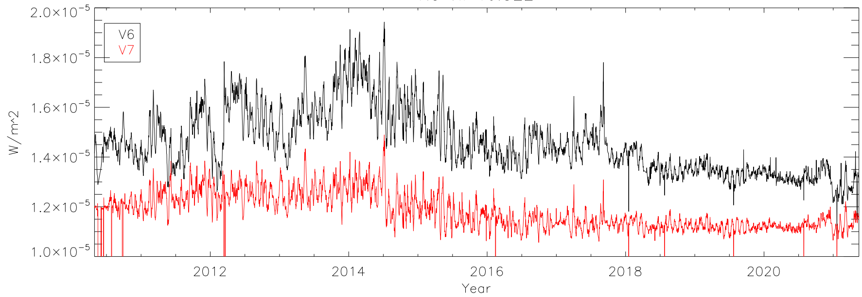
Ne VII 46.522
