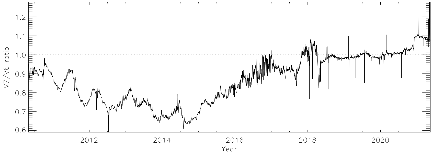
Ne VIII 77.041
