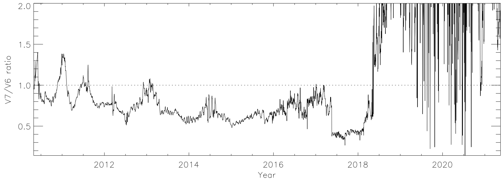
S XIV 44.570
