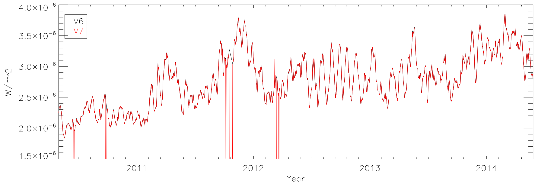
Fe VIII 13.124
