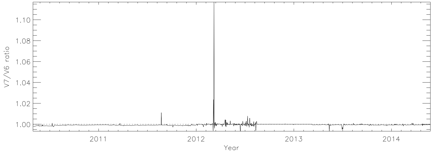
Fe VIII 13.124
