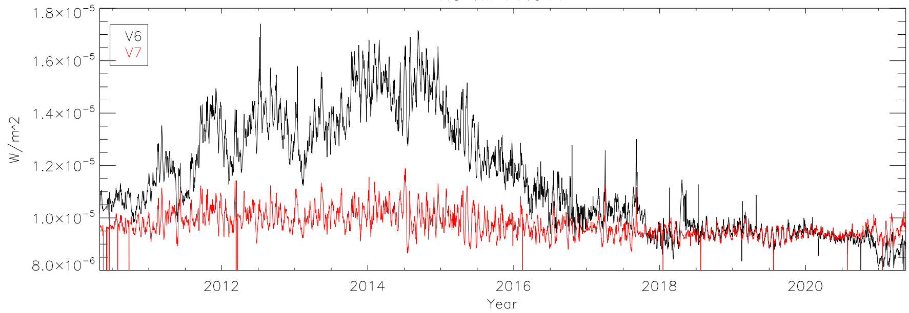
Ne VIII 77.041
