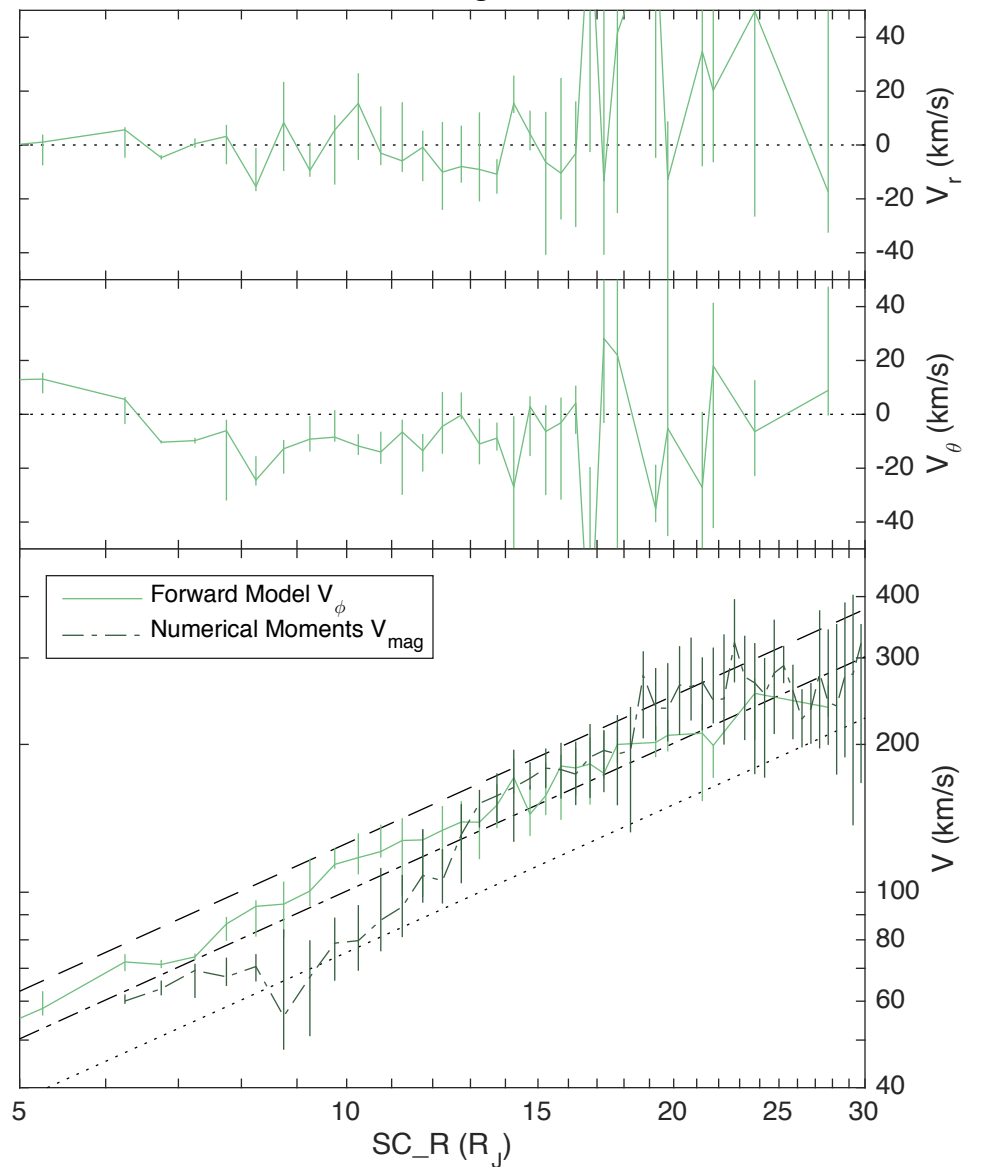
202 &lt; E. Long. &lt; 292
