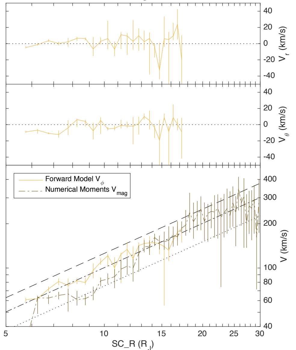
292 &lt; E. Long. &lt; 022
