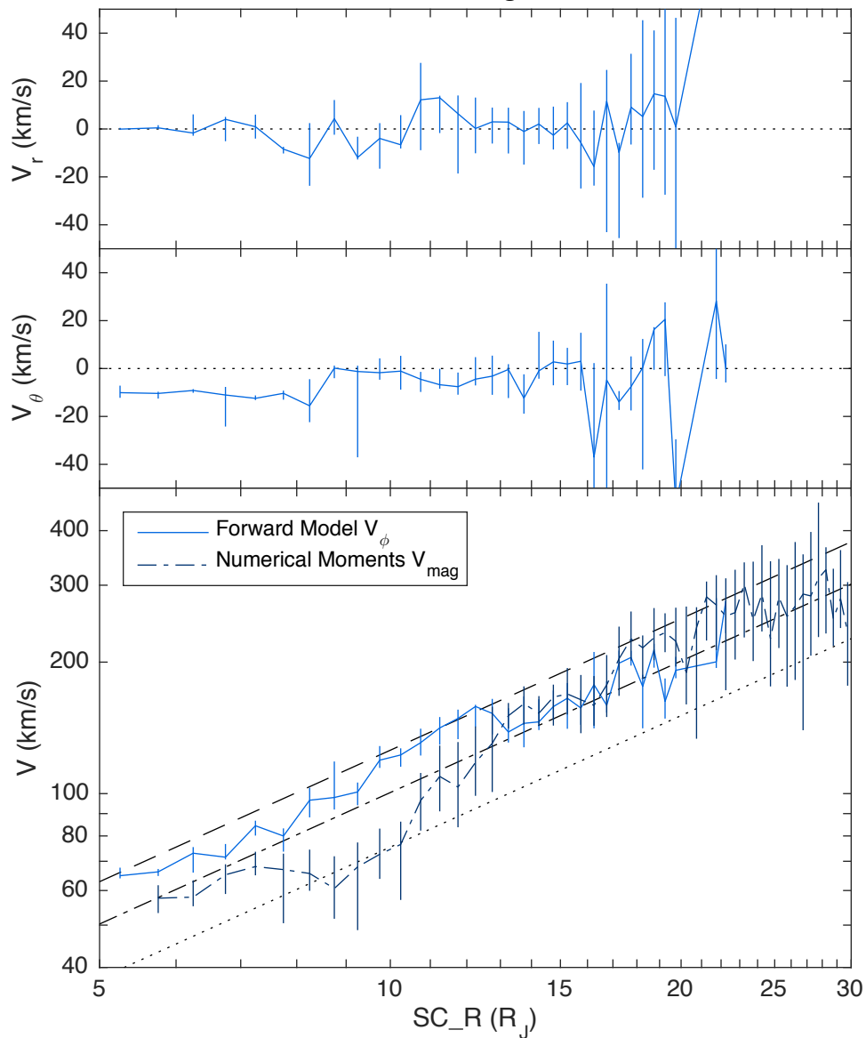
022 &lt; E. Long. &lt; 112
