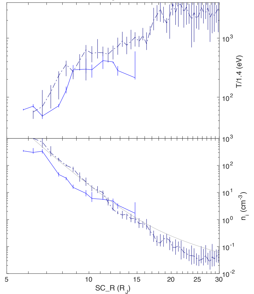
Midnight LT
