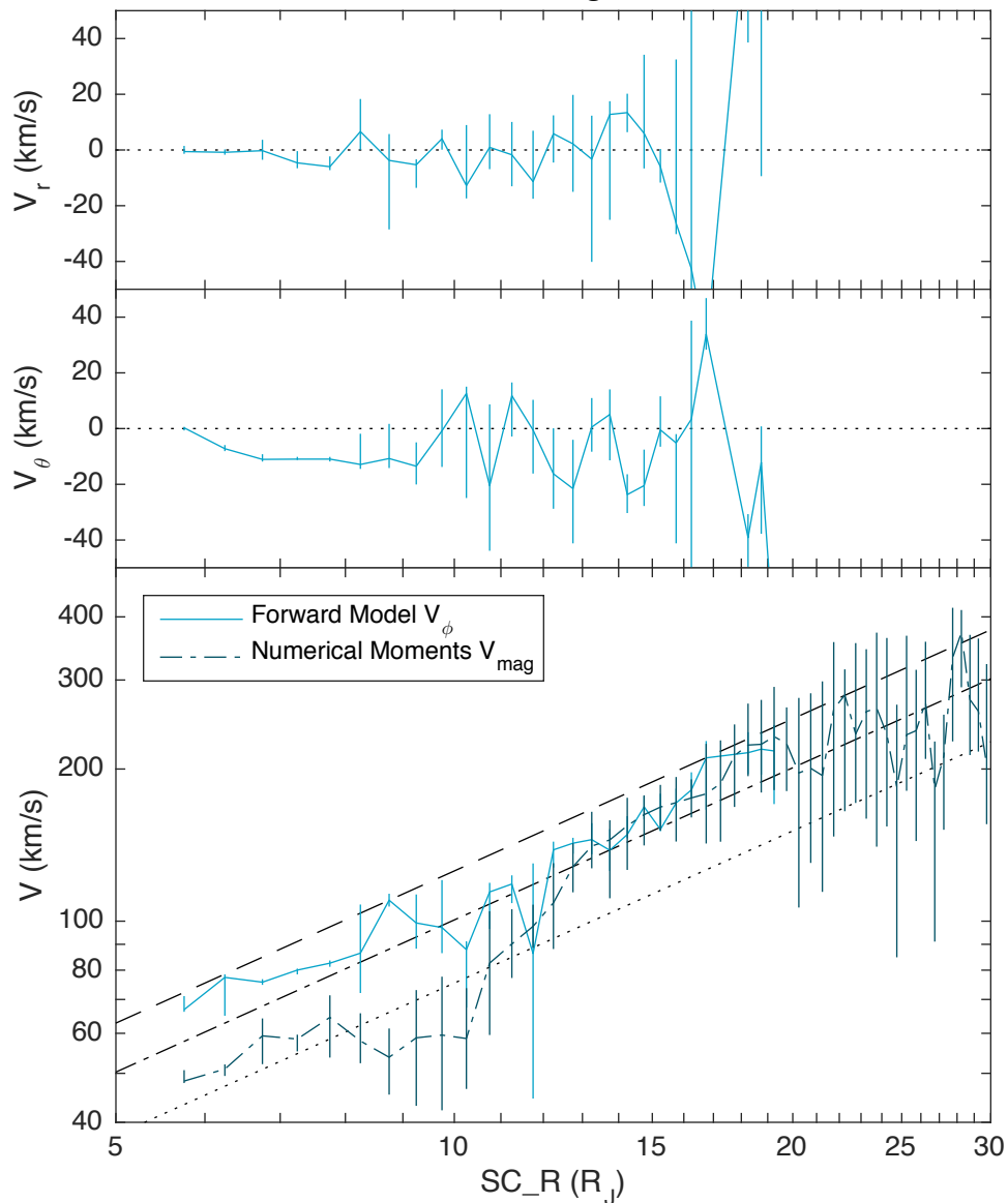
112 &lt; E. Long. &lt; 202
