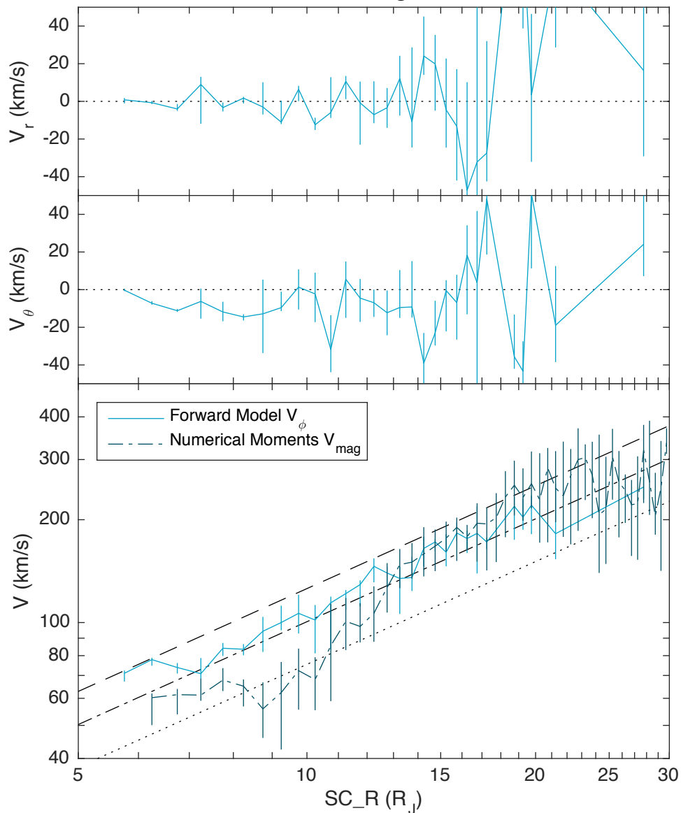
157 &lt; E. Long. &lt; 247
