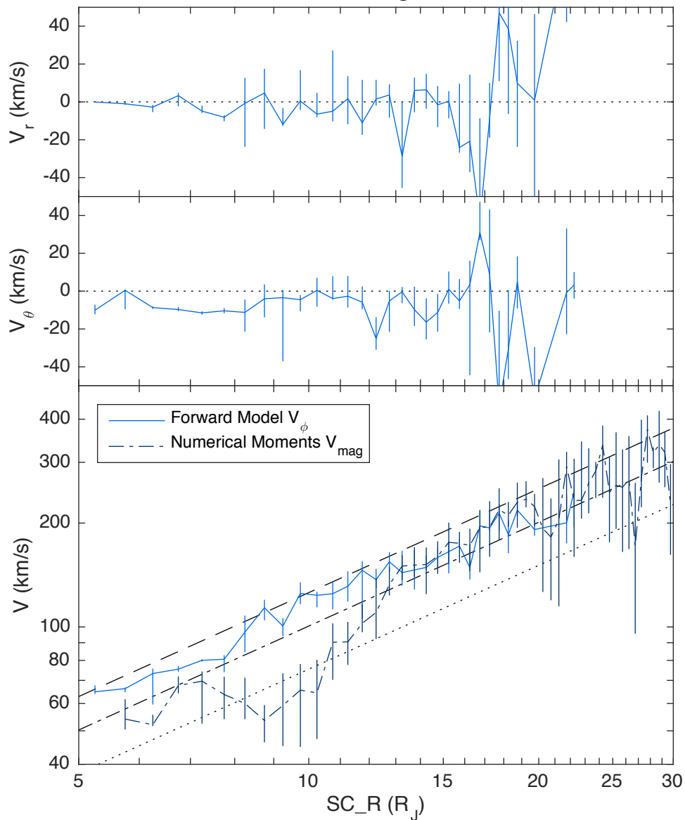
067 &lt; E. Long. &lt; 157
